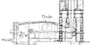
Herdovn. Smelteovn. Flammen slår over broen forbi ovdøren og stryger langs herden. Det smeltede metal aftappes t. h.
