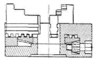
Centerpatron.
