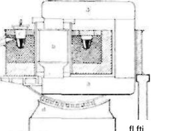
Elektroovn. Induktionsovn. a transformatorkerne, b primærvikling, c ringformet smelternde, d kippemektisme.
