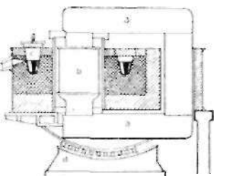
Elektroovn. Induktionsovn. a transformatorkerne, b primærvikling, c ringformet smelternde, dkippemektmisme.
